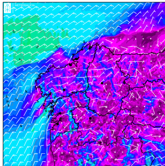
WRF ARW DET Vento 10m (km/h) 2024-01-26 12:00Z
