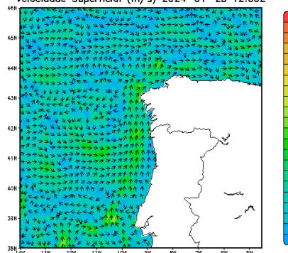
ROMS Velocidade Superficial (m/s) 2024-01-25 12:00Z
