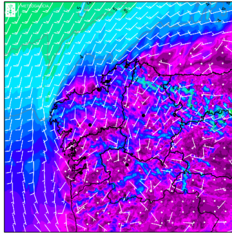
WRF ARW DET Vento 10m (km/h) 2024-01-25 12:00Z
