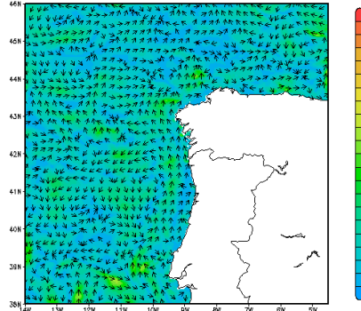
ROMS Velocidade Superficial (m/s) 2024-01-26 12:00Z
